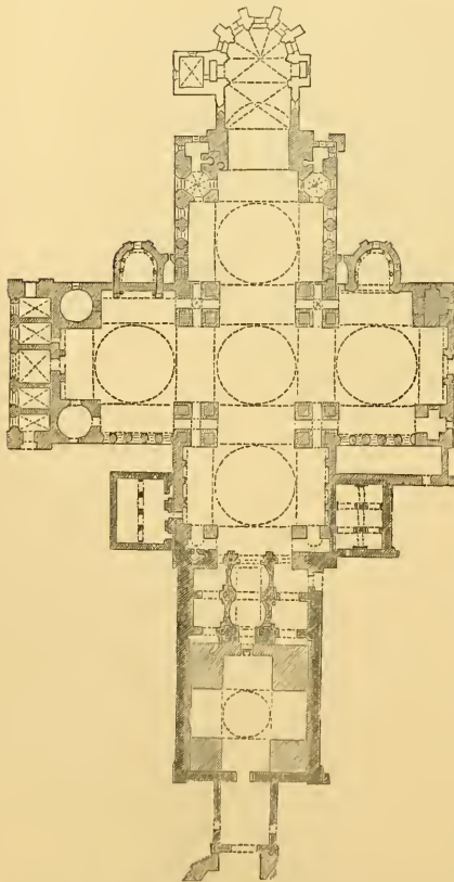
562. Plan of St. Front, Périgueux. (From F. de Verneilh, 'Architecture Byzantine en France.')
