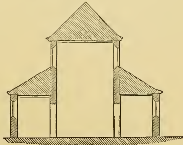
607. Plan and Section of Basse Œuvre, Beauvais. (From Woillez, 'Monuments Religieux de Beauvais.')
